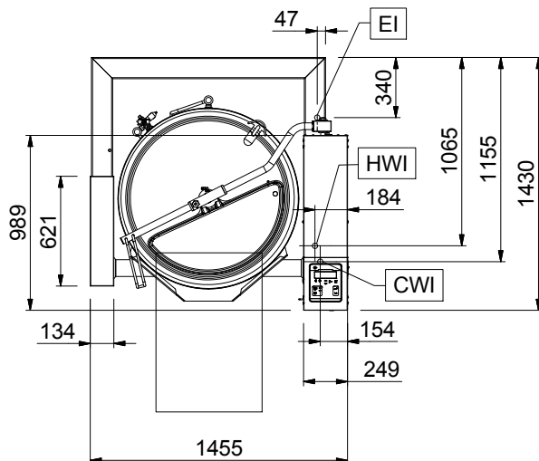
Boven aanzicht
